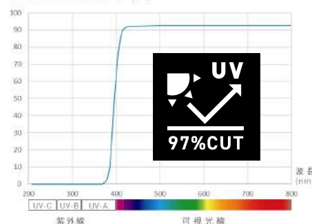
分光光線透過率(%)
